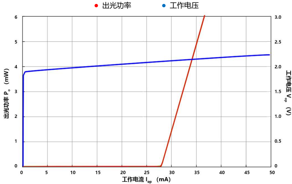
HGLD-635TO3.3-ZSP-5mW PIV 测试曲线
