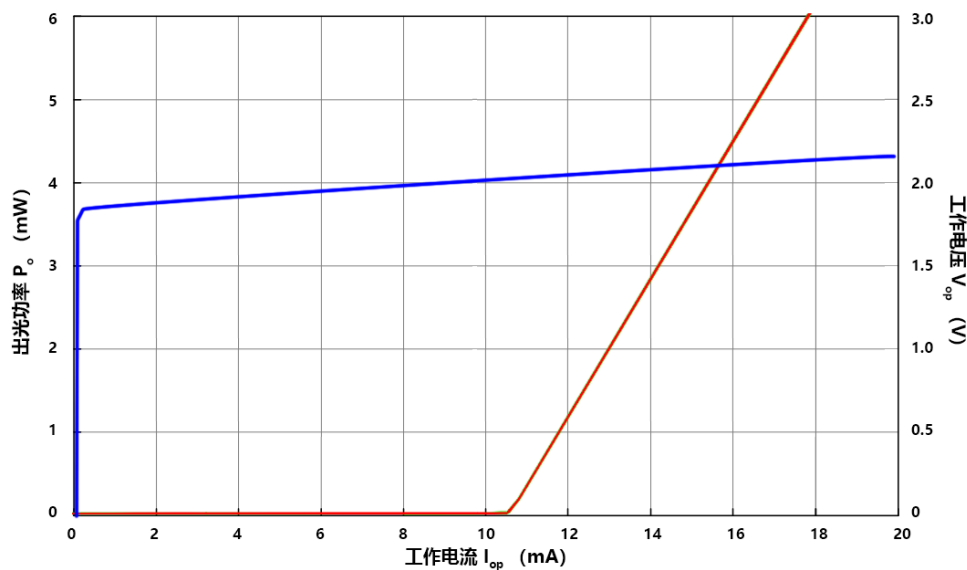
HGLD-650TO5.6-ZSP-5mW PIV 测试曲线
